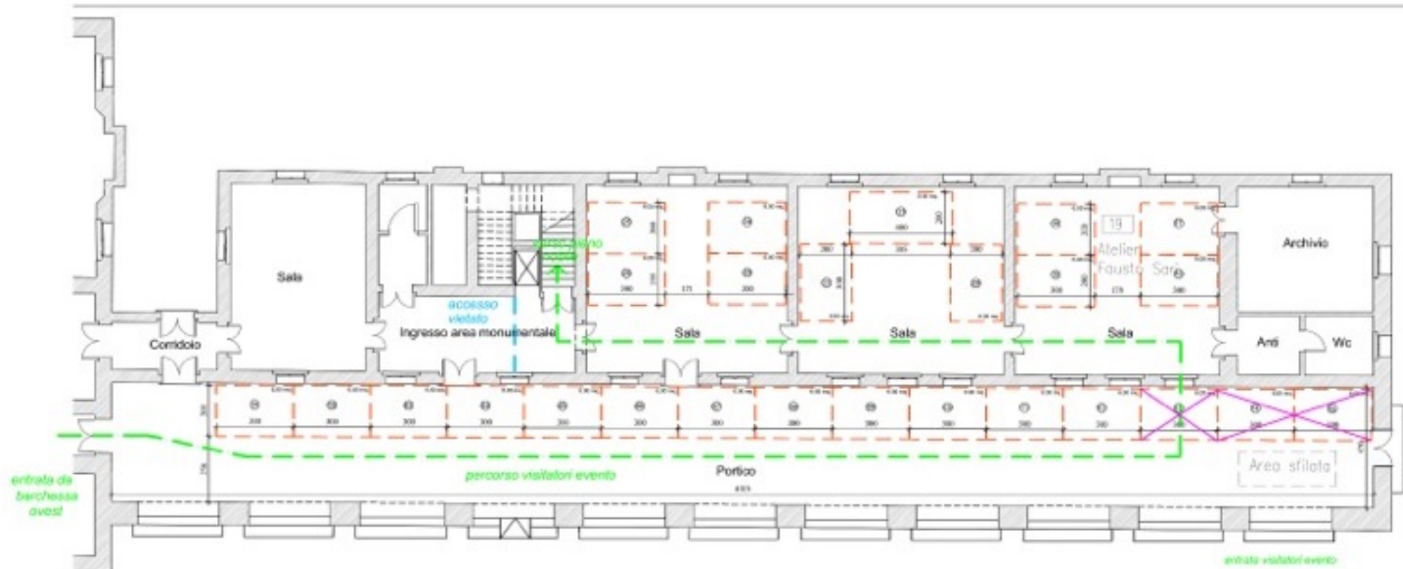
PIANO TERRA - barchessa est - Scala 1:200
